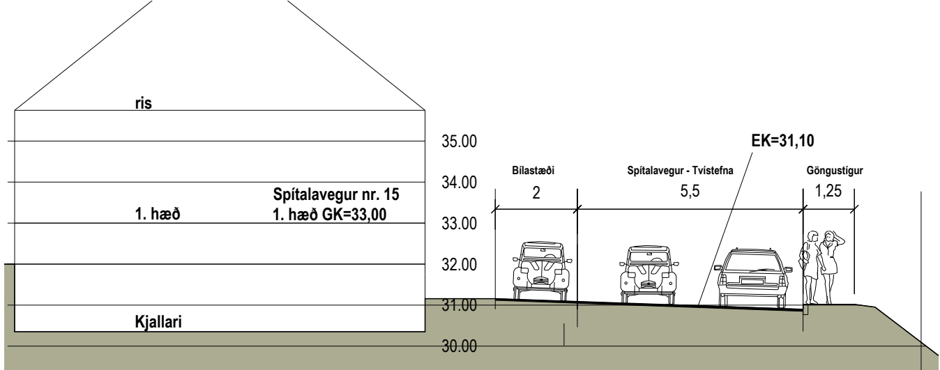
Skýringarmynd - Sníð F-F' M 1:100
