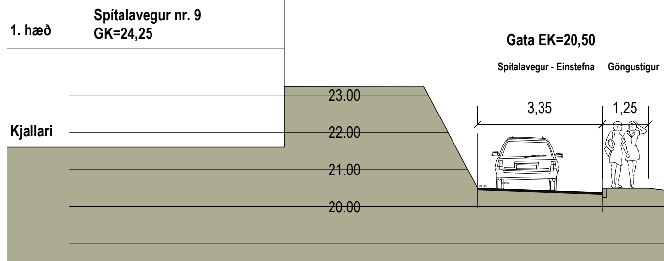
Skýringarmynd - Sníð D-D' M 1:100
