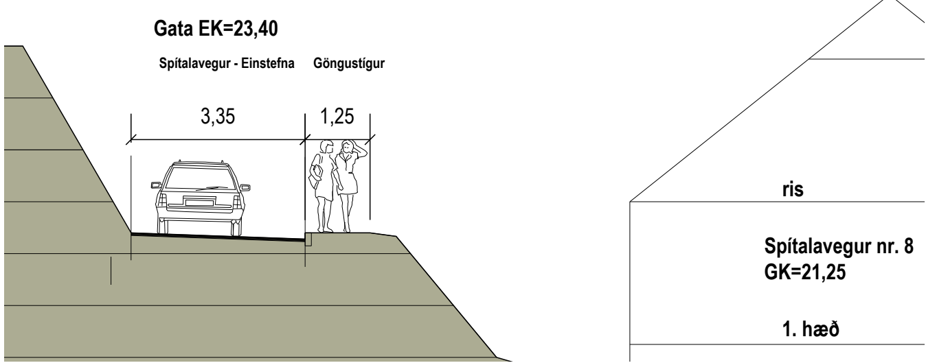
Skýringarmynd - Sníð E-E' M 1:100
