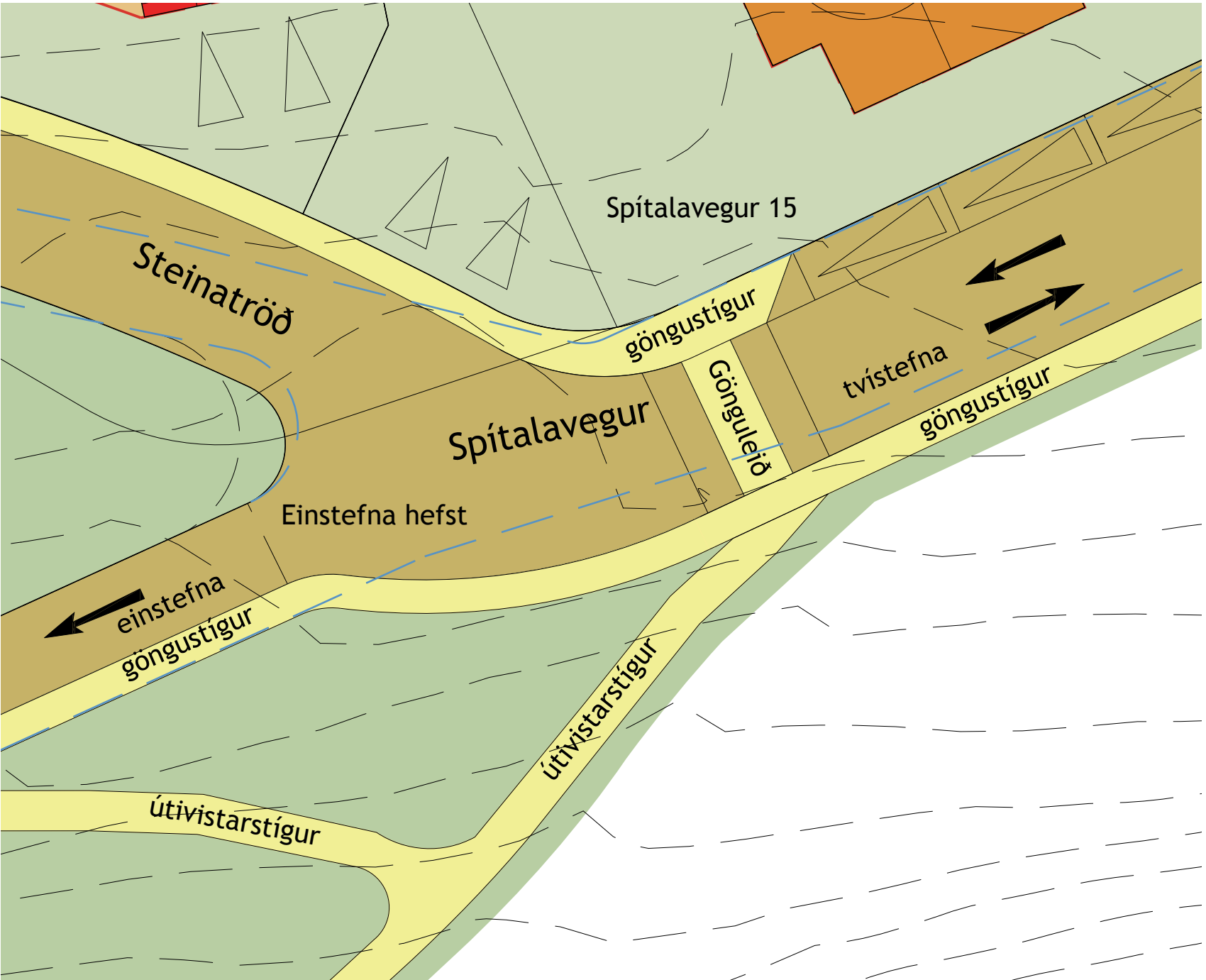
Skýringaruppdráttur - M 1:200
