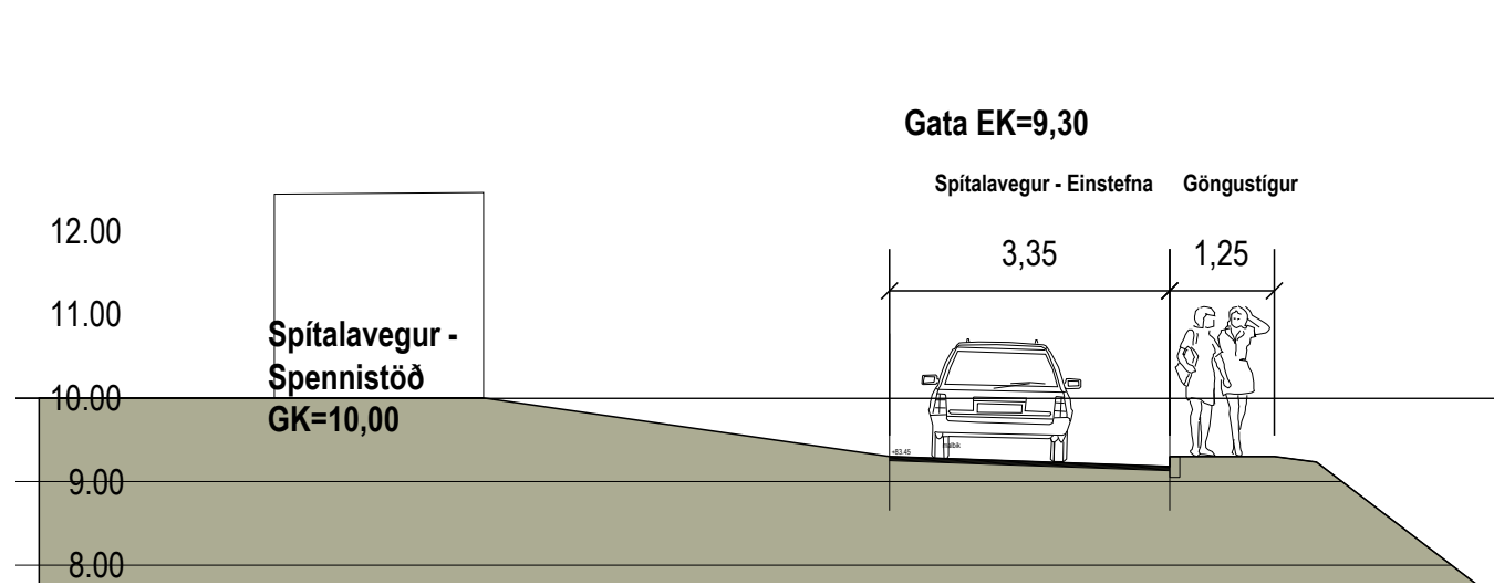
Skýringarmynd - Sníð C-C' M 1:100
