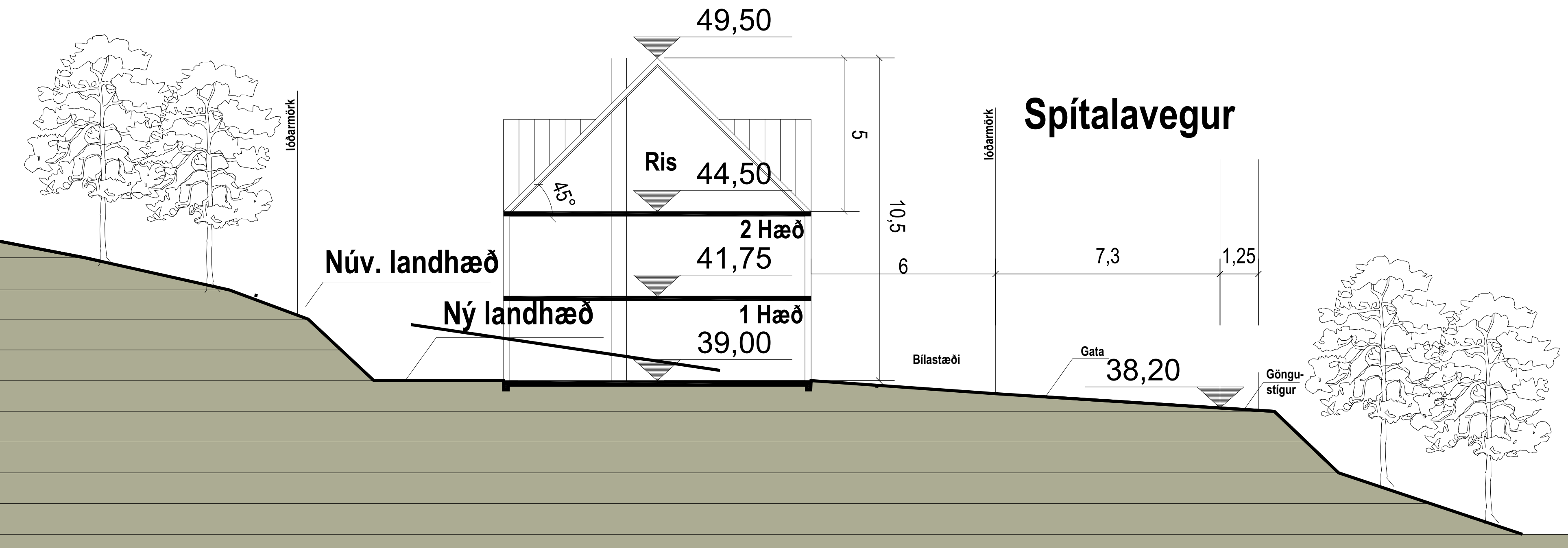
Skýringaruppdráttur Sniðteikning A - A' - Neðri hluti M 1:100
