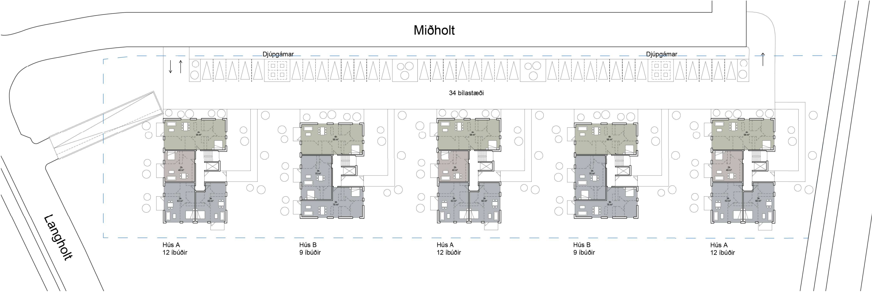
Grunmynd 1. hæðar
