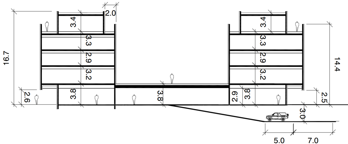
Snið - Skipagata 13
