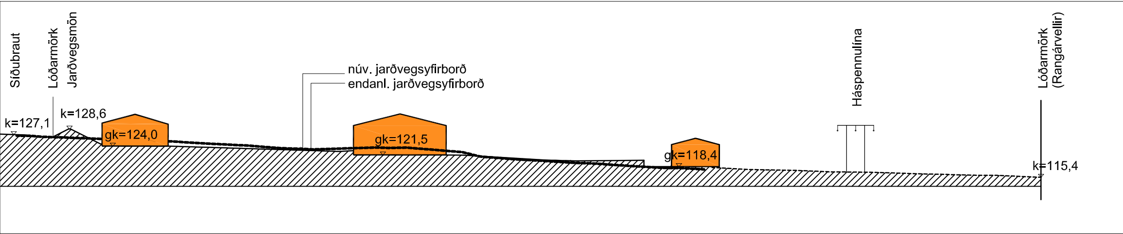
SNÍÐ A-A MKV.: 1:1000
