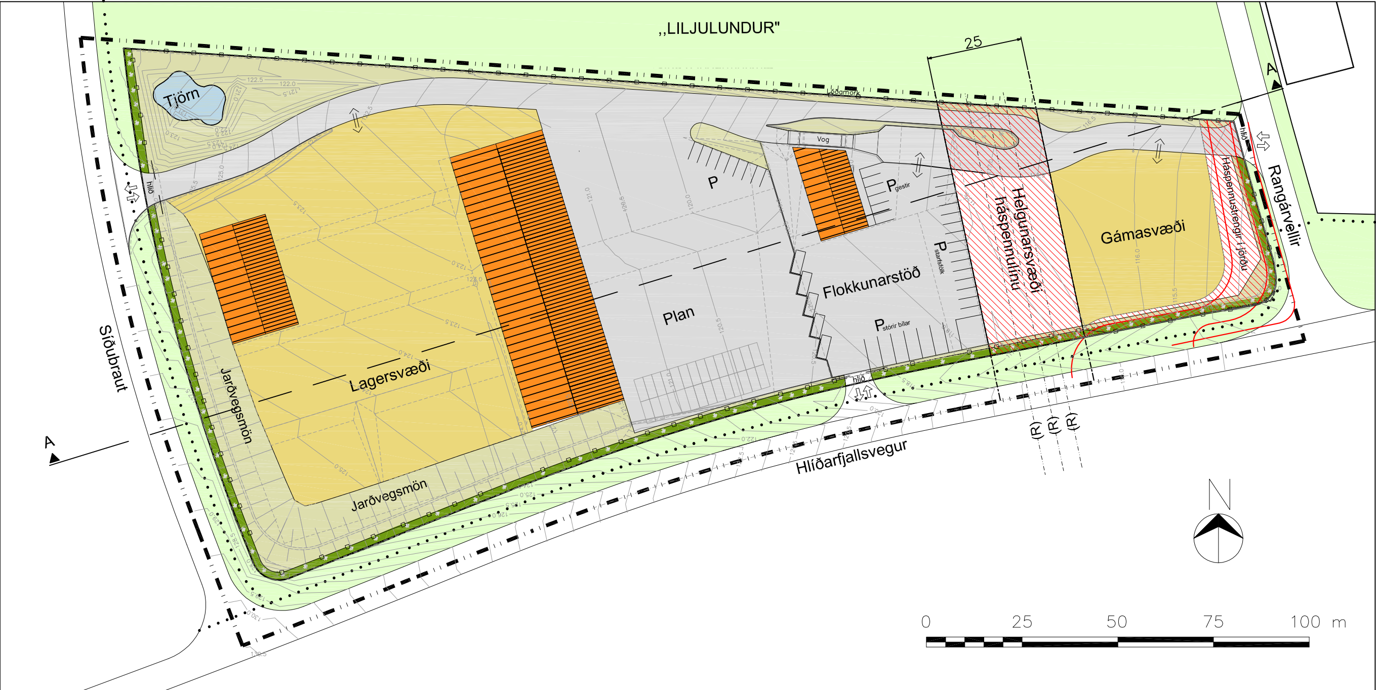
RANGÁRVELLIR, DEILISKIPULAG REITS 1.42.10 I (ASAK 2005-2018 m.s.b.) MKV.: 1:1000 Eftir breytingu
