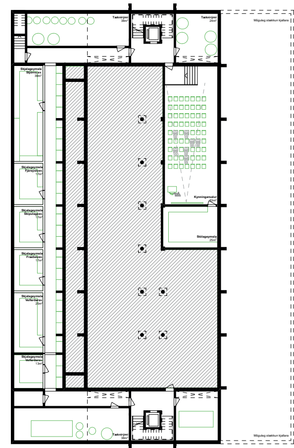
Grunnmynd Kjallari
