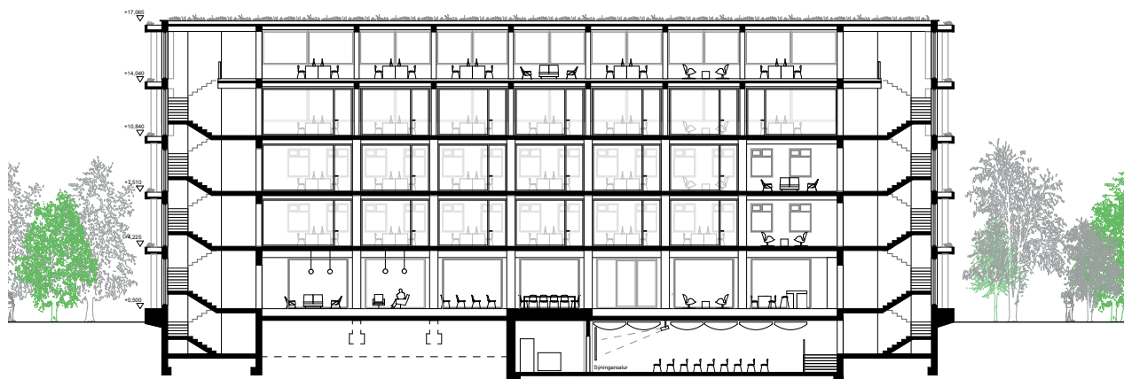
Langsnið B-B
