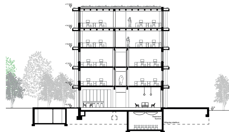
Þversnið A-A
